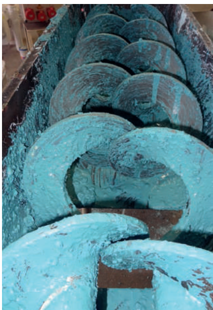
Dvojitý bezosý spirálový dopravník pro dopravu extrémně lepkavých materiálů
